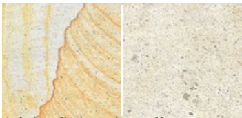
Dácittufa / Dacite tuff
