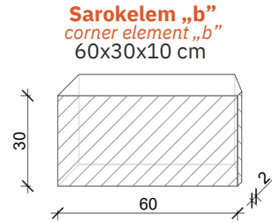
Sarokelem „b” + Sarokelem „c” + Falazó elem corner element „b” + corner element „c” + masonry element
